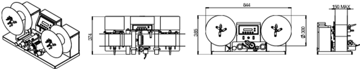
Abmessungen JR-300 Basic
