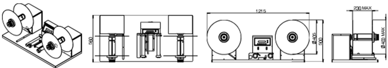
Abmessungen JR-400 JUMBO
