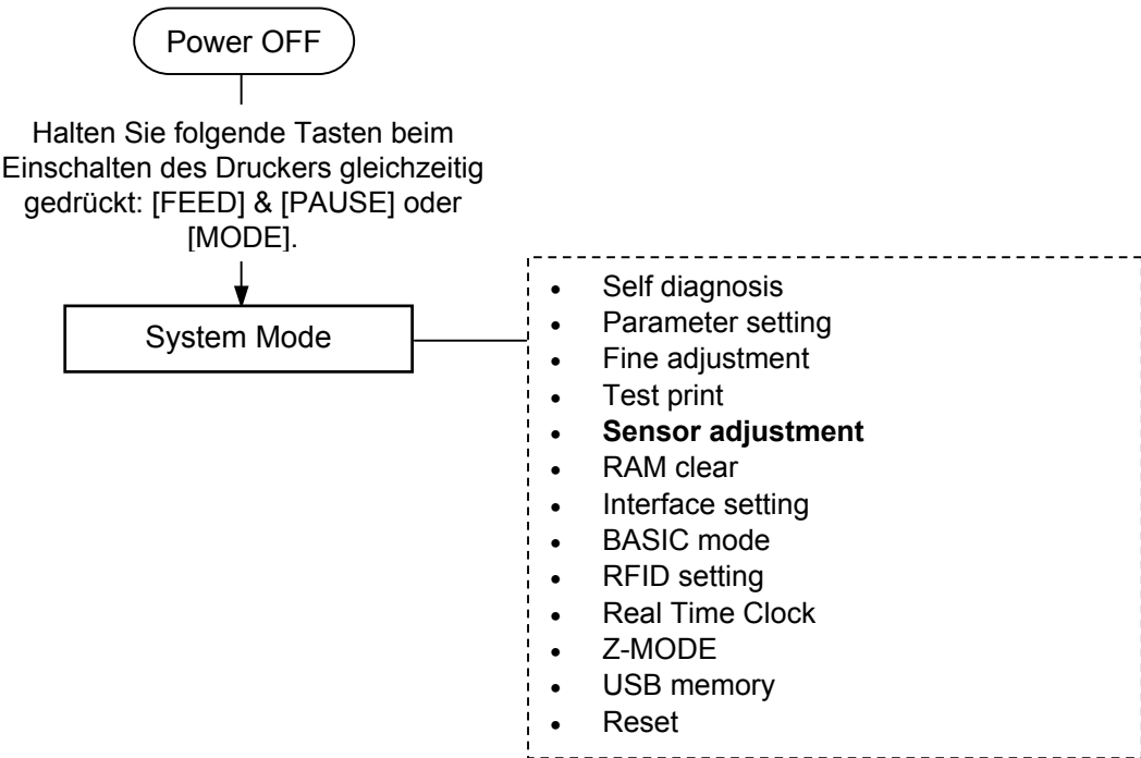
Inhalt des Sensor Adjust Menu
