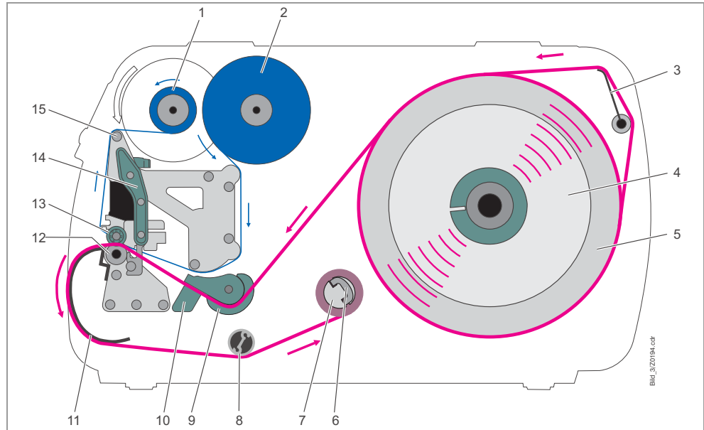
[2] Material- und Folienverlauf im AP 5.4 mit internem Aufwickler.
