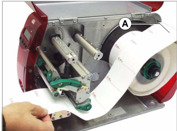
[5] Etikettenmaterial einlegen.
