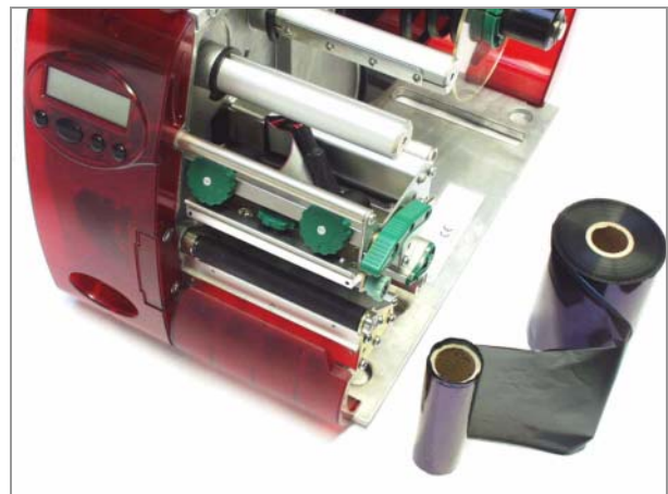
[17] Folienrollen paarweise aufbewahren.
