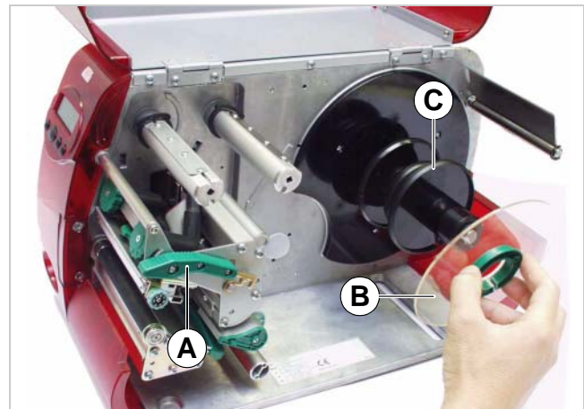
[4] Materialabroller am AP 5.4.
