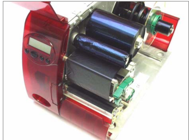
[15] AP 5.4 mit eingelegter Folie, Anruckhebel geöffnet.
