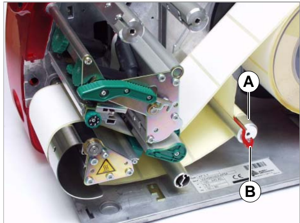
[9] Materialverlauf im AP 5.4 mit internem Aufwickler.
