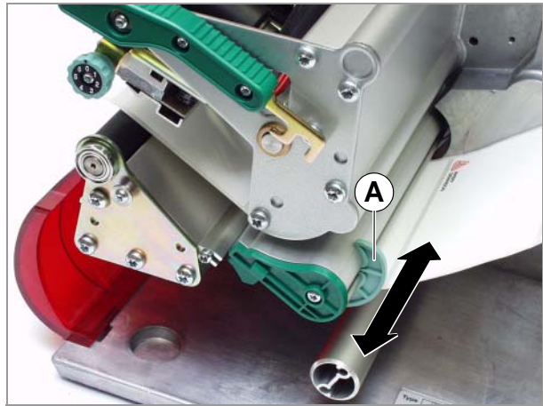
[6] Materialführung (A) einstellen.
