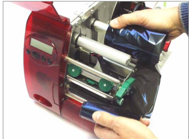
[16] Beide Rollenrollen abziehen.
