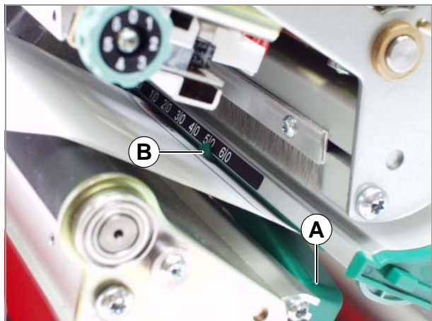
[7] Etikettenlichtschranke einstellen.
