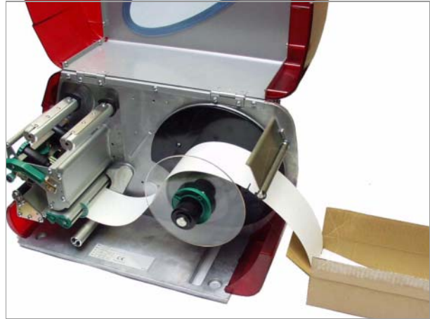
[8] Leporello-Material einlegen.
